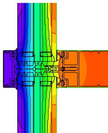
Izotermický priebeh
