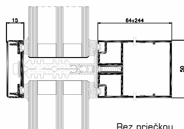
Rez priečkou
